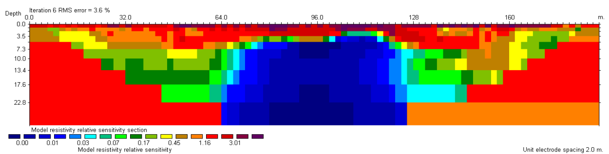
Figure 2 : Haut, panneau électrique interprété (dispositif pole-dipole) de 190 m de long avec un écartement inter électrode de 2m. Bas, carte de sensibilité de l'inversion, avec un minimum au niveau de la zone très résistante.
